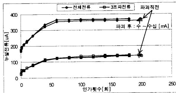
(b) 8/20 [ \mu\text{s} ] 인가시
