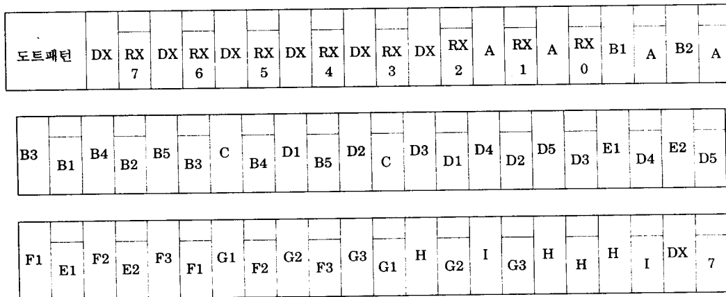
그림 3-1. 전송 시퀀스의 천이
