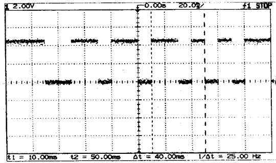
그림 4-7. DSC 신호의 파형(일부분)
