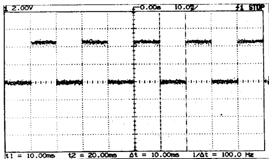
그림 4-6. 200비트 비트패턴의 신호파형
