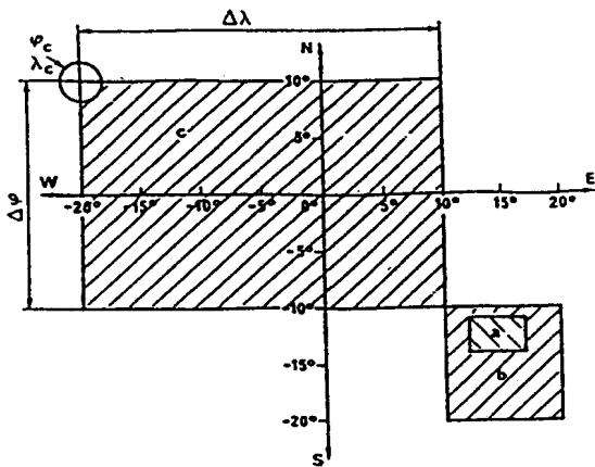
그림 3-2. 지리적좌표
