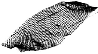
Fig. 9 Rolling mode (13.28 Hz)
