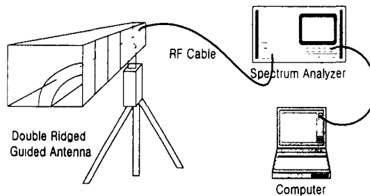
그림 4. 전파측정 시스템의 전체 구성도
