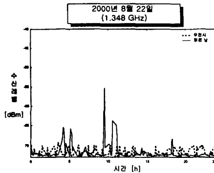
그림 24. 맑은 날과 강우일의 비교 특성
