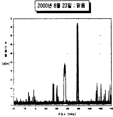
그림 9. 아침시간대(06:00 - 08:00)의 측정데이터
