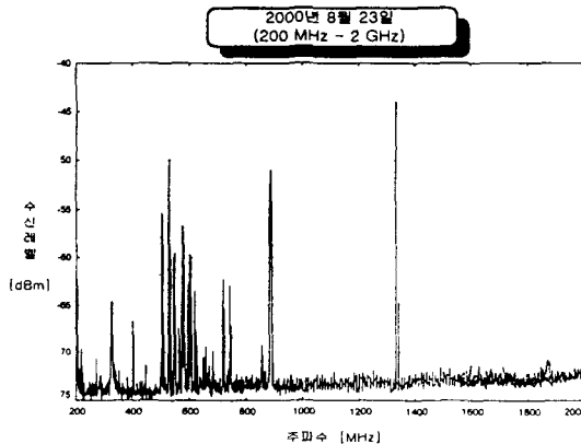
그림 8. 측정 데이터 (방송)
