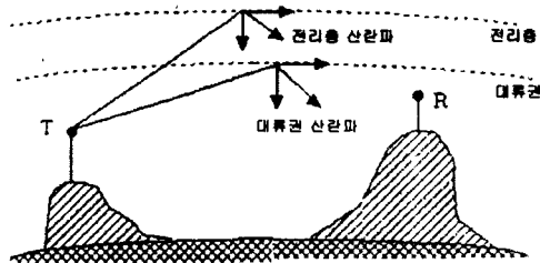
그림 2. 대류권 산란에 의한 전파 전파
