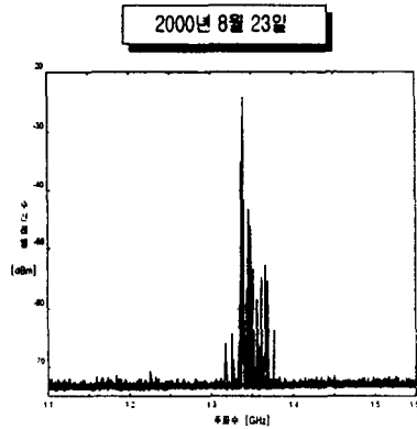
그림 19. 저녁시간대(18:00~20:00)의 측정 데이터
