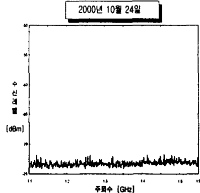
그림 21. 우천시의 측정 데이터
