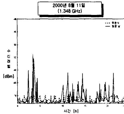
그림 23. 맑은 날과 강우일의 비교 특성
