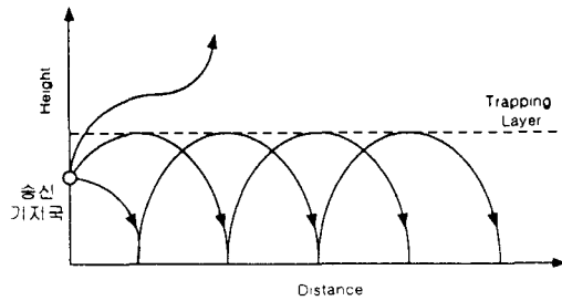
그림 3. 덕팅 전파 전파
