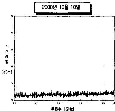
그림 20. 맑은 날의 측정 데이터
