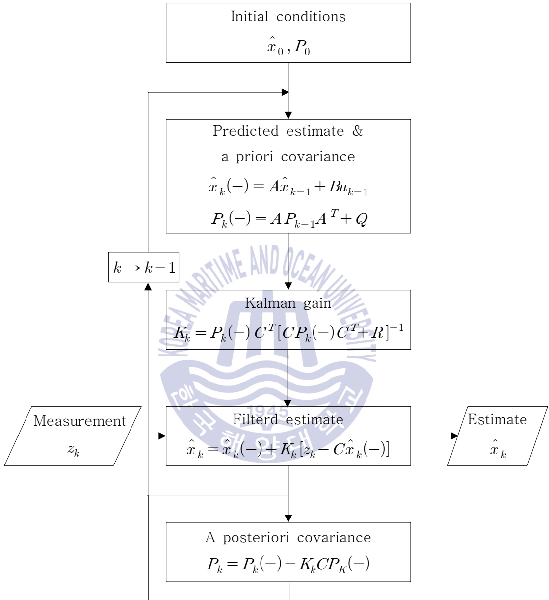
그림 3.1 Kalman 필터 알고리즘 계산 흐름선도
